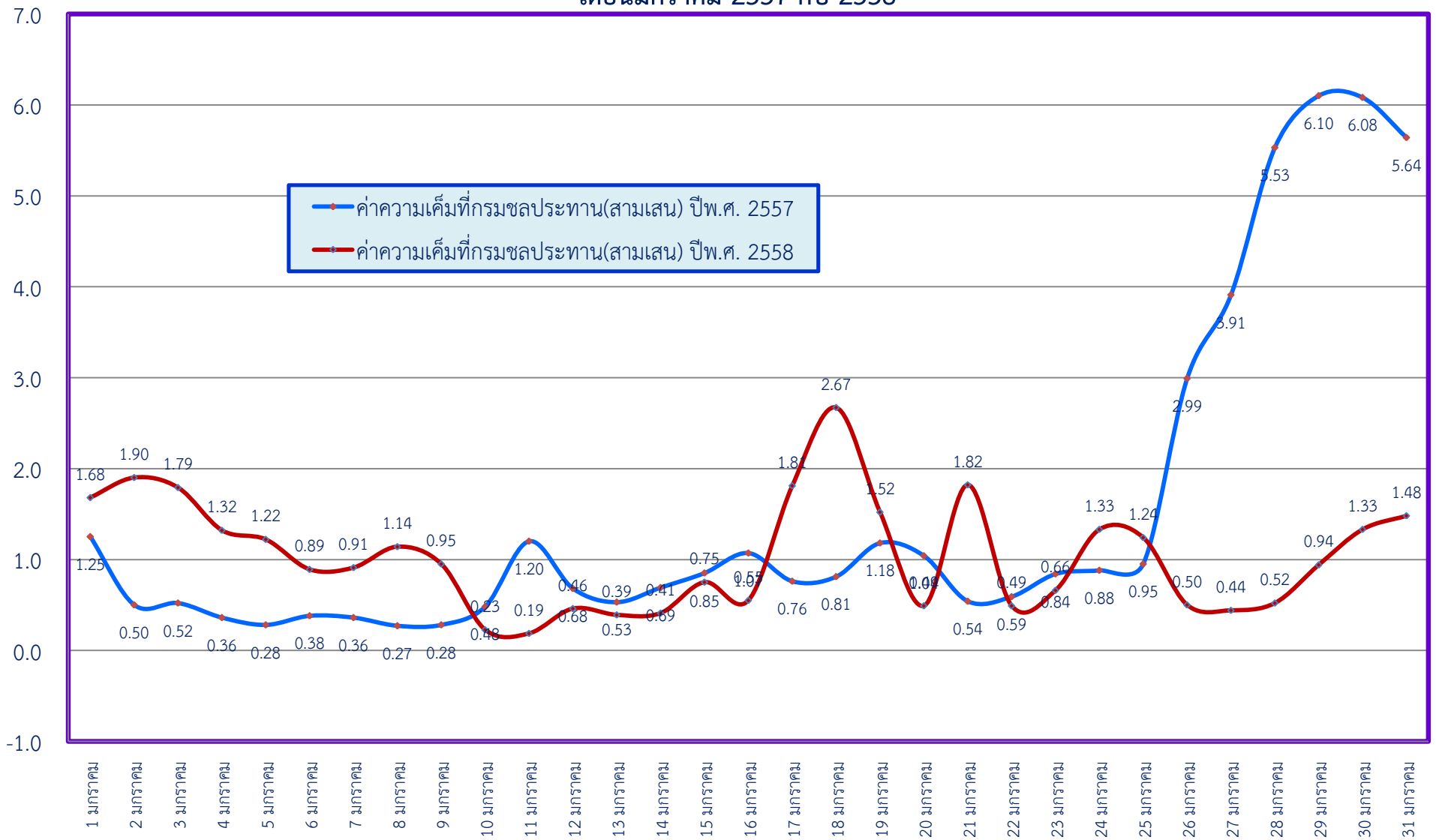
กราฟแสดงการเปรียบเทียบค่าความเค็มในแม่น้ำเจ้าพระยา ที่จุดตรวจวัดกรมชลประทาน(สามเสน) เดือนมกราคม 2557 กับ 2558
